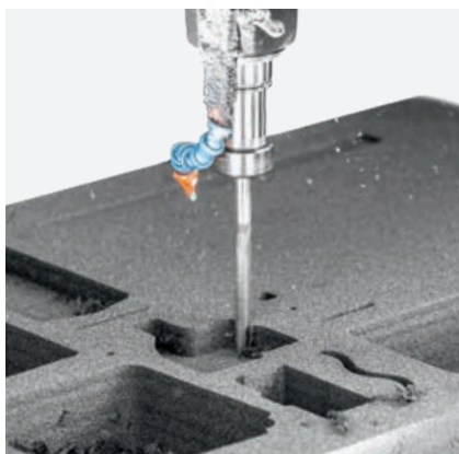
Nauwkeurige bewerking met waterstraalmachine of de CNC-freesmachine
